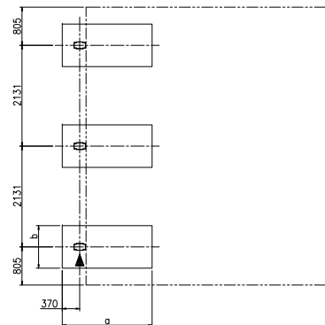
柱・基礎位置図 (S = 1 / 50) ▶: 排水位置を示す
