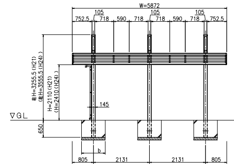
側面図 (S = 1 / 50)
