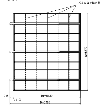
平面図 (S = 1 / 50)
